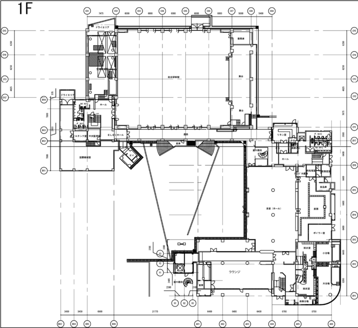
厨房平面図
